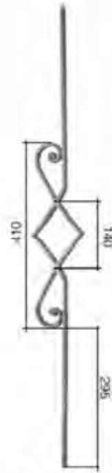
Art. 302A03 \square 14X8mm H.1000 mm L.100 mm
