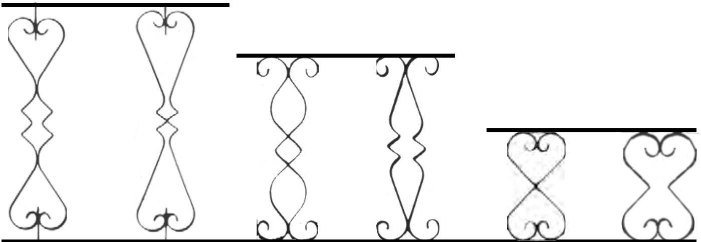
49A19 \square 20x4 49A22 \square 20x4 49A25 \square 20x4 49A28 \square 20x4 49A31 \square 20x4 49A34 \square 20x4 49A20 \square 25x4 49A23 \square 25x4 49A26 \square 25x4 49A29 \square 25x4 49A32 \square 25x4 49A35 \square 25x4 49A21 \square 30x4 49A24 \square 30x4 49A27 \square 30x4 49A30 \square 30x4 49A33 \square 30x4 49A36 \square 30x4 H 800 mm H 800 mm H 550 mm H 550 mm H 350 mm H 250 mm
