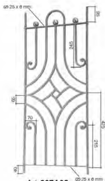
Art. 307A02 \varnothing 12 mm H.1000 mm L. 420 mm
