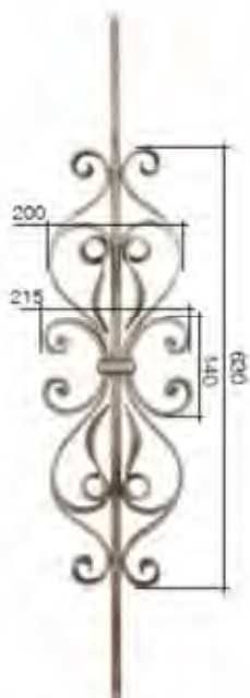
Art. 304A04 \phi 14 mm H.1000 mm L. 215 mm
