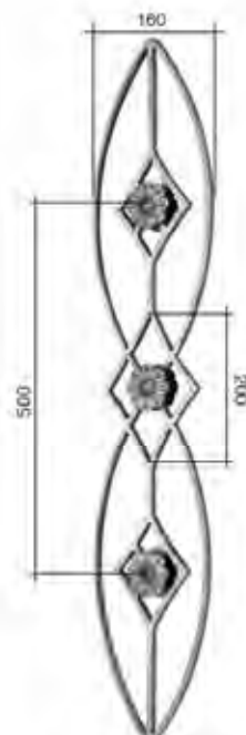
Art. 303A02 \square 14X8mm H.1000 mm L.190 mm
