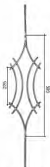
Art. 302B06 \varnothing 12 mm H.1000 mm L. 200 mm
