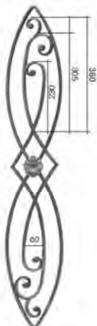
Art. 303A01 \square 14X8mm H.1000 mm L.190 mm
