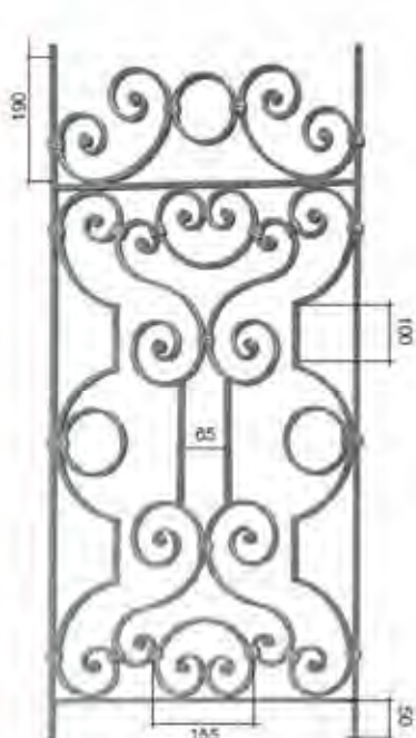
Art. 312A06 ∅14 x 8 mm H. 1000 mm L. 475 mm
