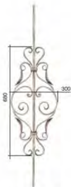
Art. 304A01 \phi 14 mm H.1000 mm L. 300 mm
