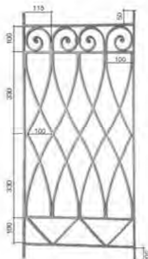
Art. 311A02 ∅14 x 8 mm H.1000 mm L. 480 mm
