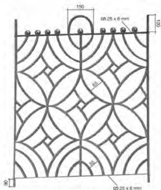
Art. 307A01 \varnothing 12 mm H.1000 mm L. 830 mm
