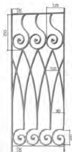
Art. 311A03 ∅14 x 8 mm H.1000 mm L. 395 mm
