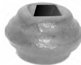
Art. 177B17 Ø 37 H 25 Foro □ 12 Art. 177B18 Ø 40 H 25 Foro □ 14 Art. 177B19 Ø 55 H 35 Foro □ 20 Art. 177B20 Ø 55 H 35 Foro □ 22 Art. 177B22 Ø 70 H 35 Foro □ 25 Art. 177B23 Ø 70 H 35 Foro □ 30
